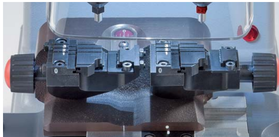
Etaux basculants (0° +/- 45°) avec 3 emplacements du mise en place clé
