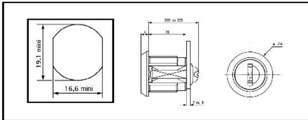
BAT-7308-B9B Cam de type 72-73
