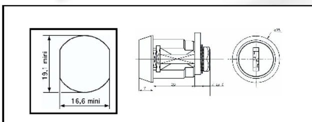
Réf : BAT-7416-B3B Cam de type 72-73
