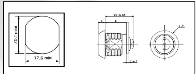
BAT-7303-B9B Cam de type 72-73
