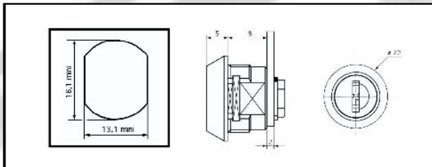
Réf : BAT-7150-B68B Cam de type M2
