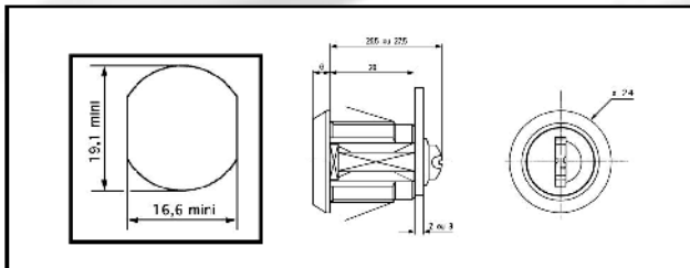
BAT-7360-B76B Cam de type 72-73
