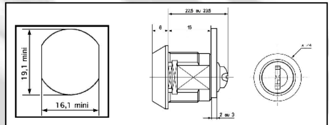
BAT-7310-B16B Cam de type 72-73
